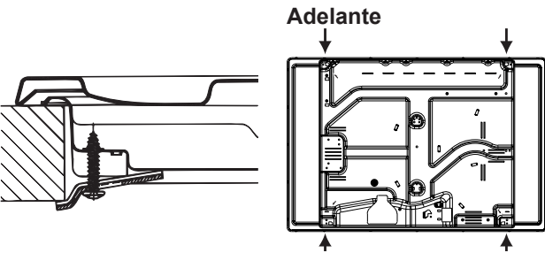
Posición del gancho para superficies H=40mm
