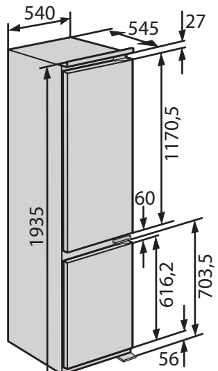
CB 20 M
