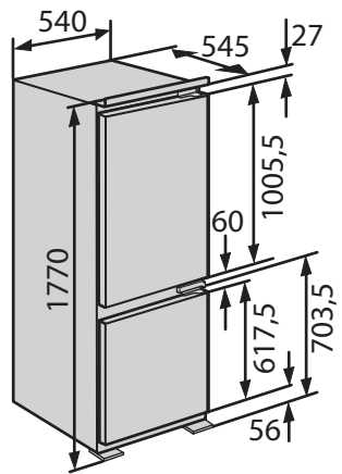
CB 18M 70/30
